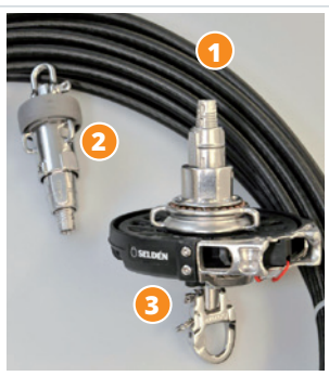
Das Seldén-GX Komplett-Kit beinhaltet:
